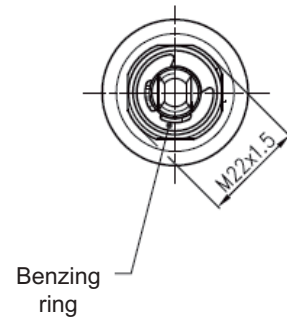
P3 pin
